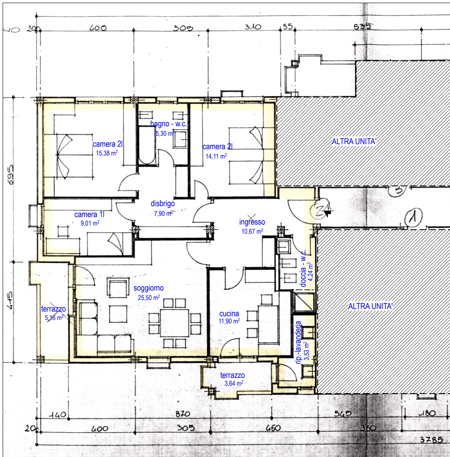
piano secondo
